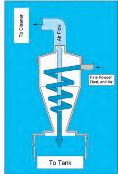
Centrifugal Action of Mini Porter Cyclone
